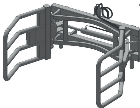
PINCE BALLE HYDRAULIQUE APPB-180 CF
