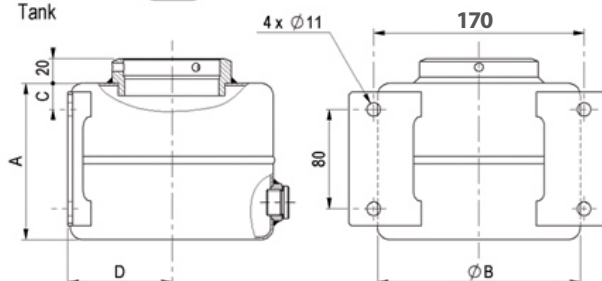
Réservoir Reservoir Tank
